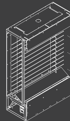
FLEXOTRAP® L1
